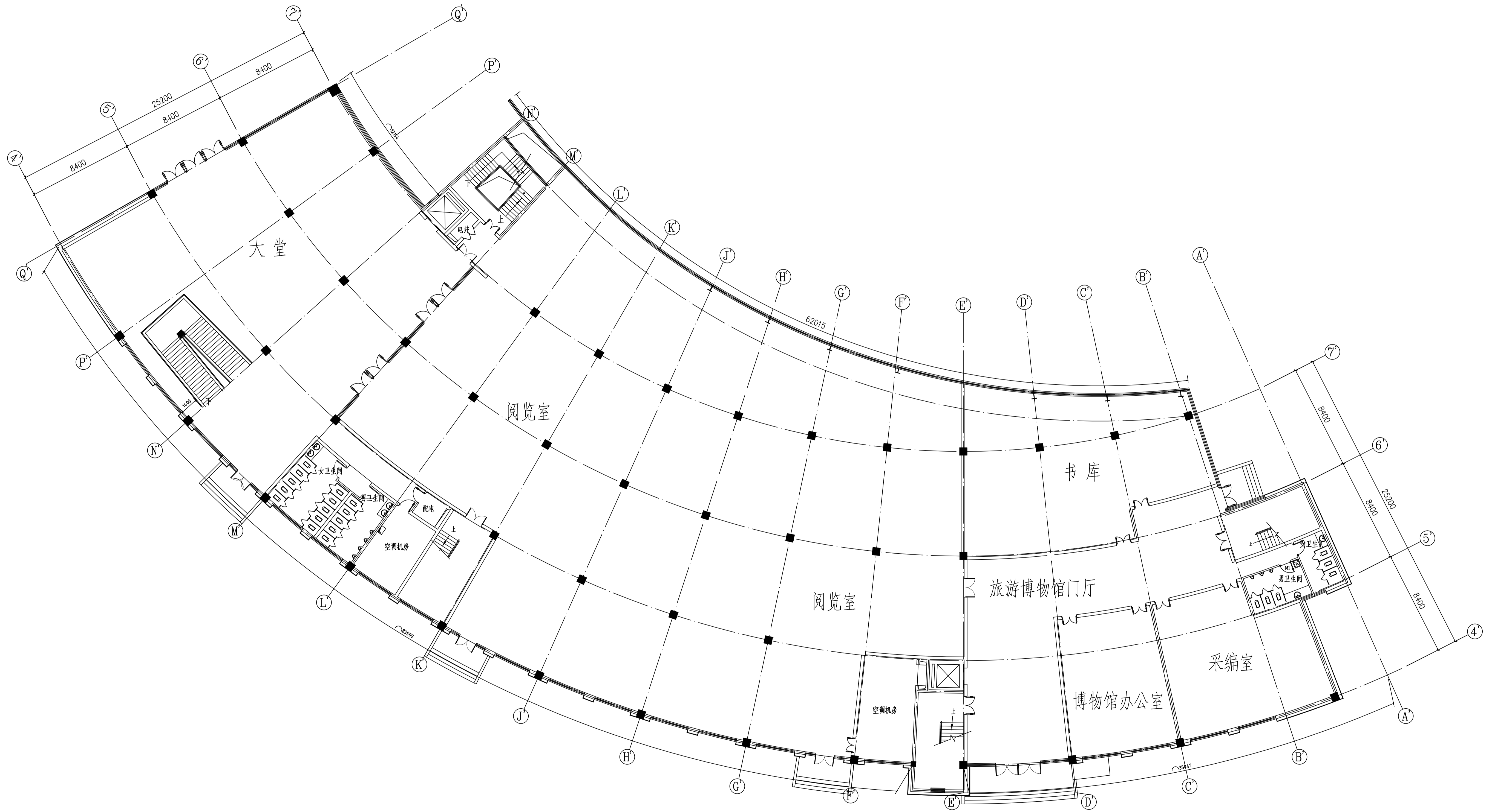
图书馆一层平面图 建筑面积: 3042.9m 2
