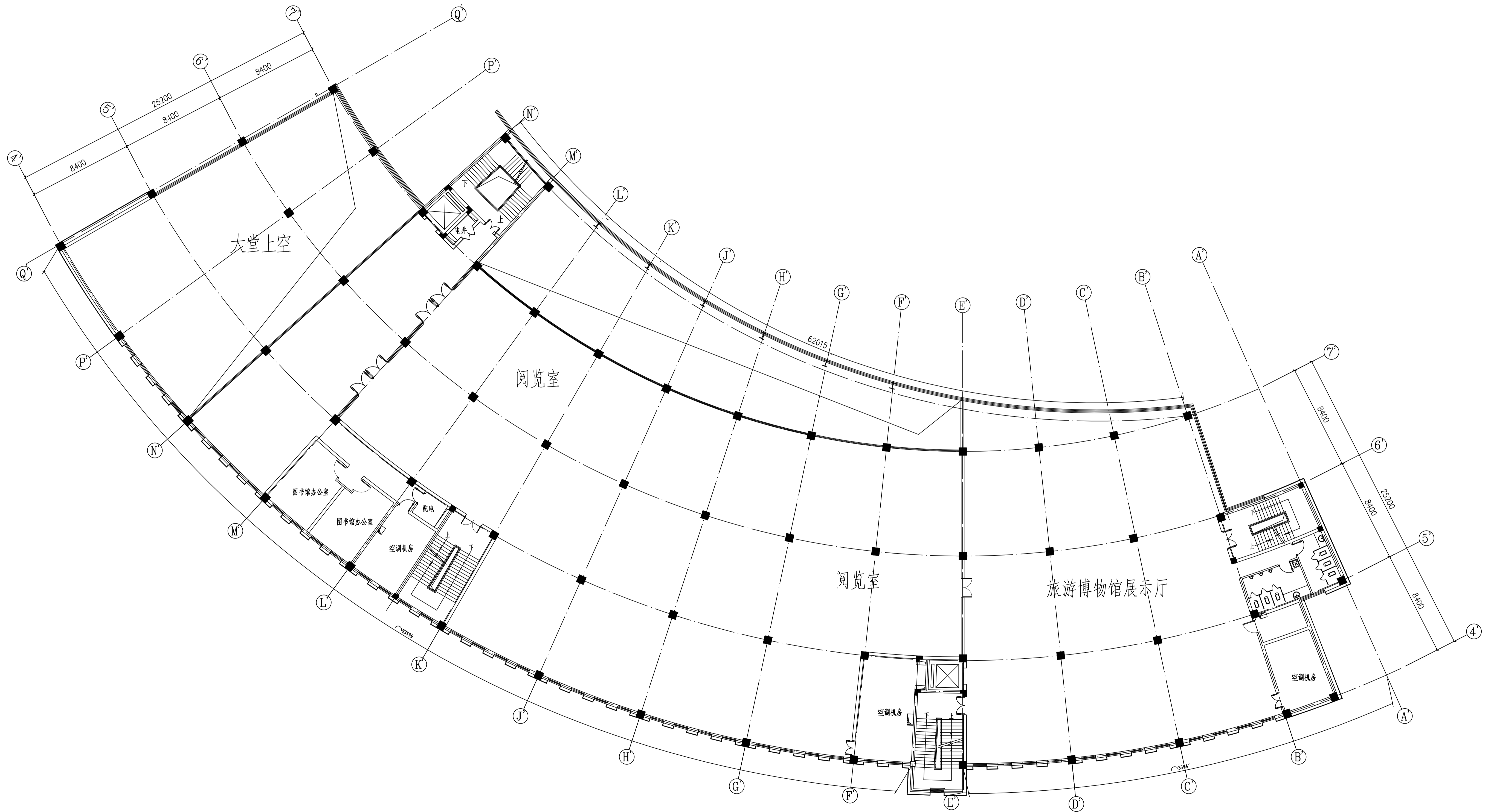
图书馆三层平面图 建筑面积: 2260.8m 2
