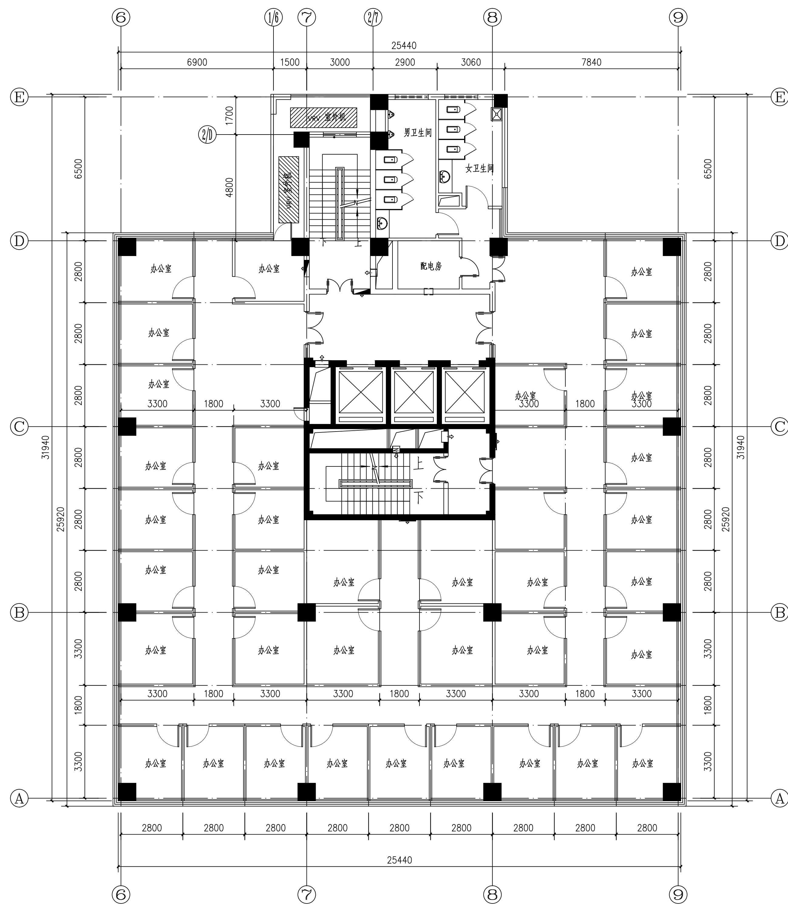
教授工作室平面图 1:100
