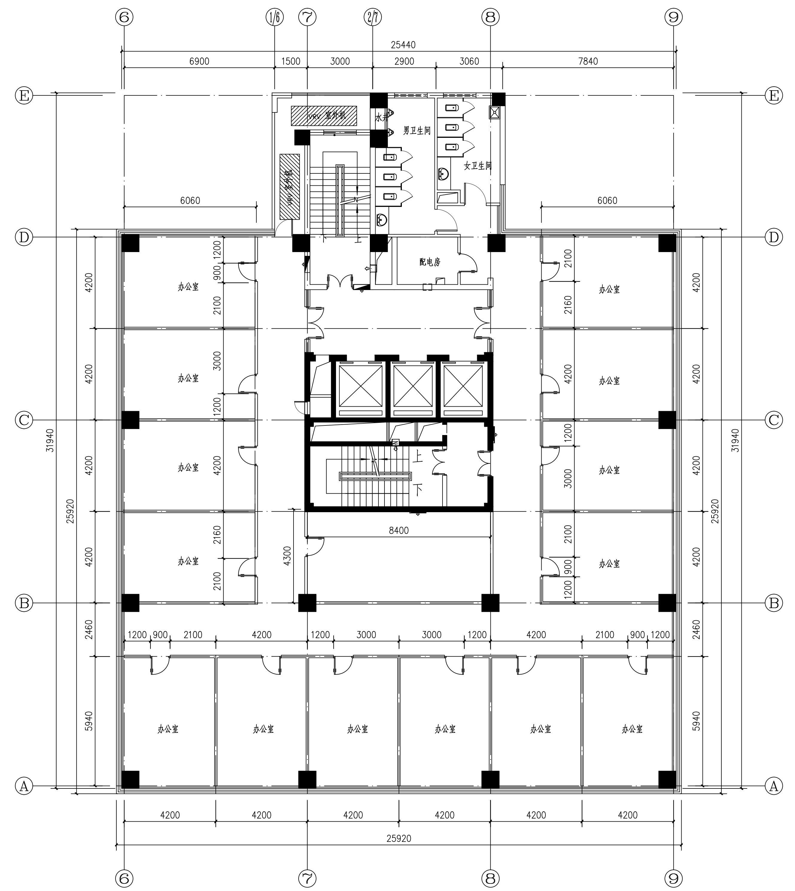
标准层平面图 1:100
